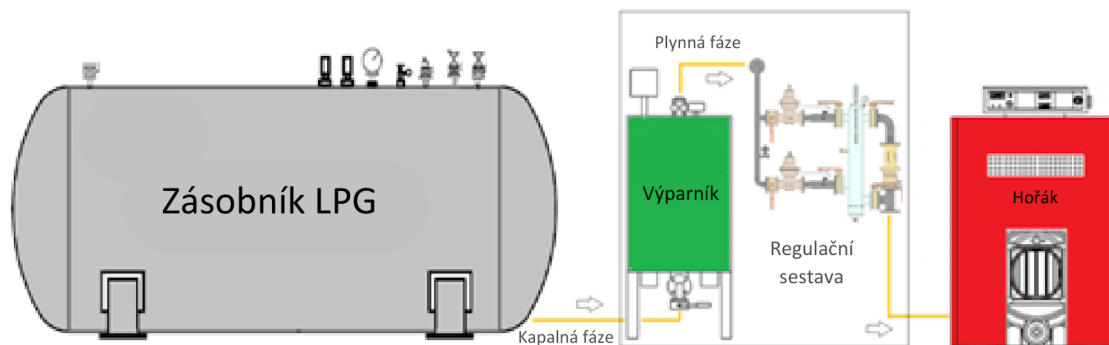
obr.: Zapojení výparníkové stanice
